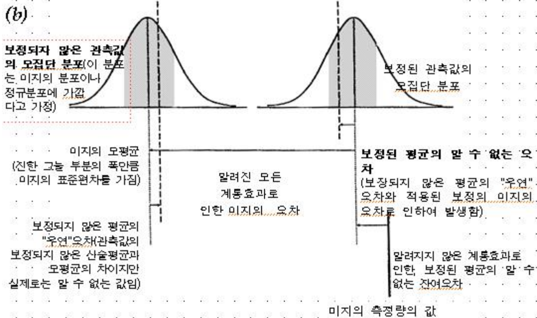
그림 1.1 오차와 불확도의 개념
