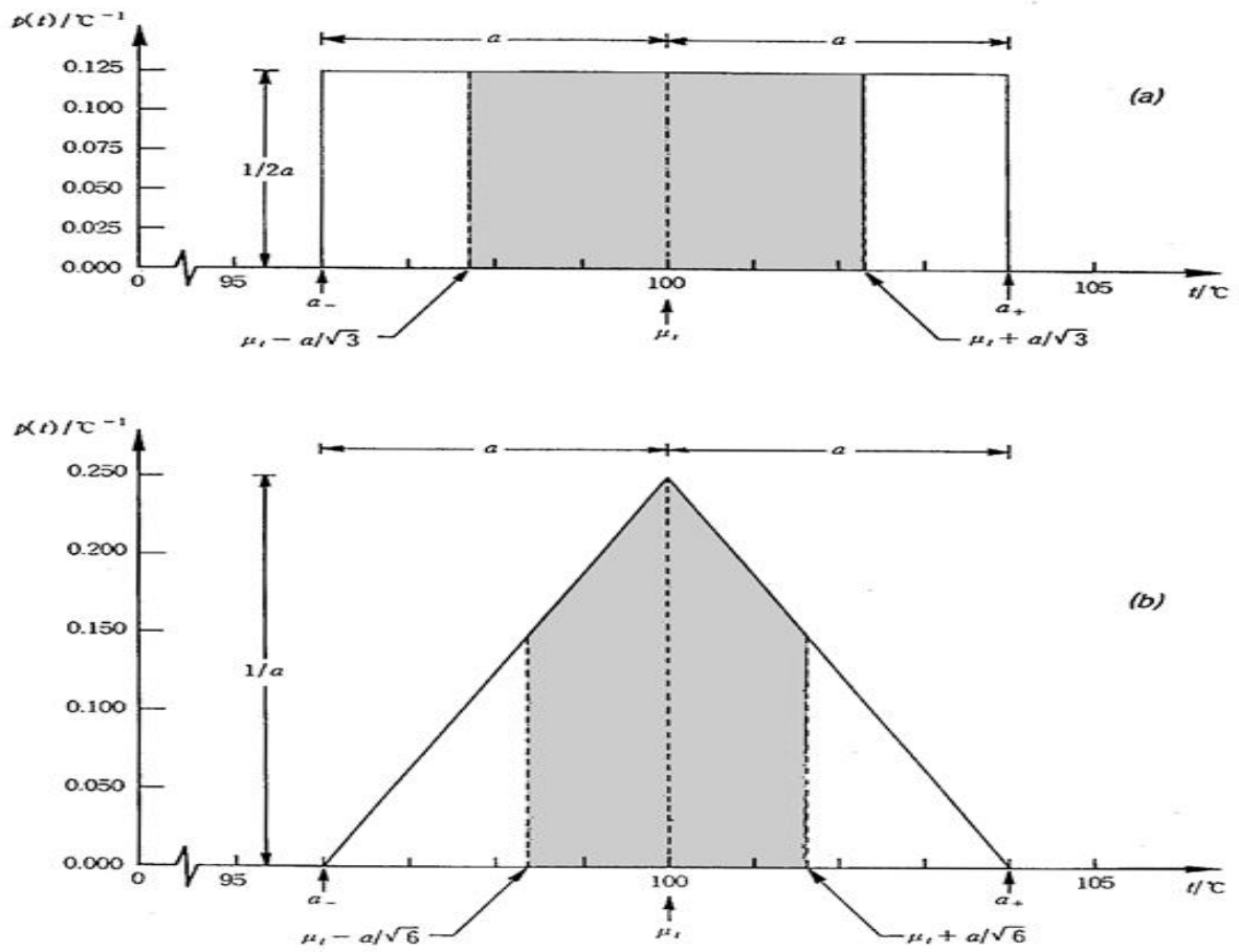
그림 2.2. 선형적 분포로부터 얻은 입력량의 표준불확도 평가
