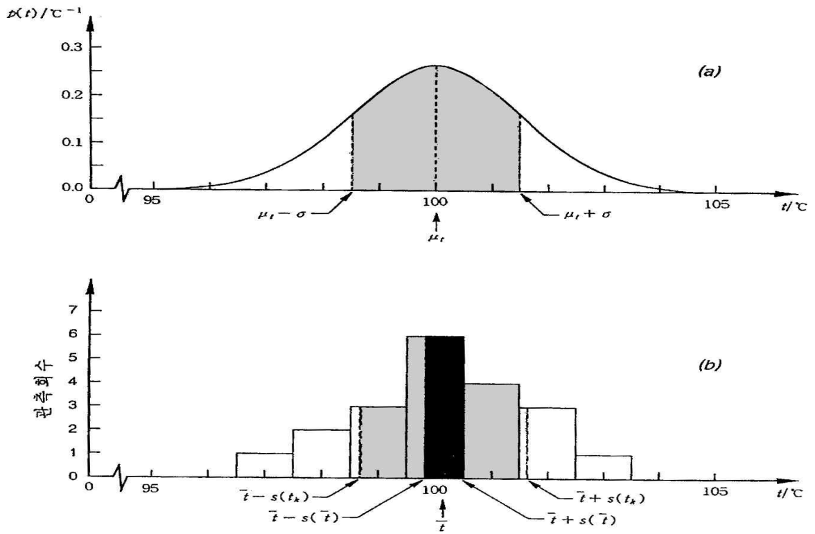
그림 2.1. 반복된 관측으로부터 얻은 입력량의 표준불확도 평가
