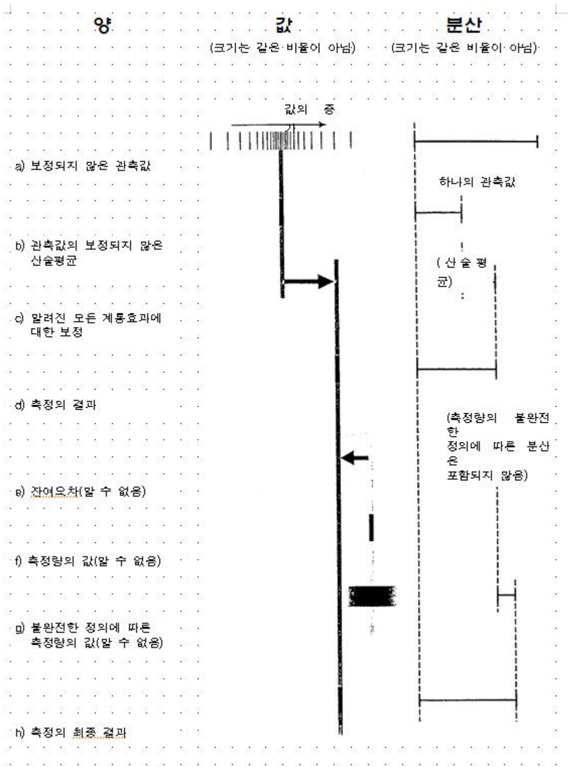
그림 1.2 값, 오차, 불확도의 개념
